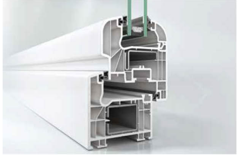
Schüco CT 70 Rondo
