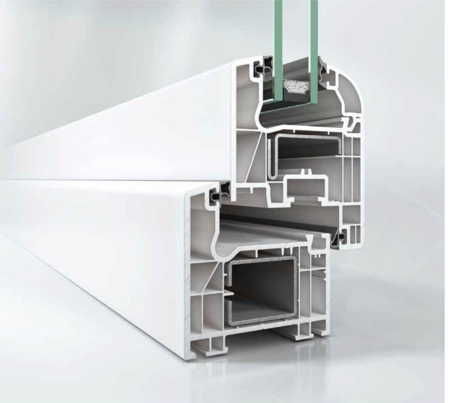
Schüco CT 70 Classic
